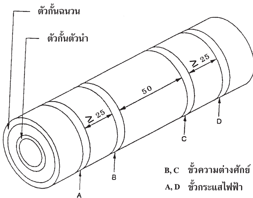
รูปที่ 6 การทดสอบความต้านทานของตัวกันฉนวน (ข้อ 10.16.3.1 และข้อ 10.16.3.4)
