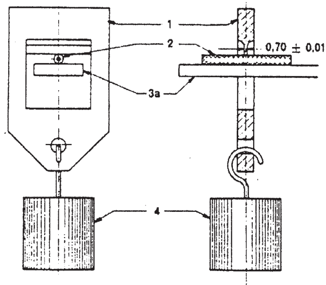
รูปที่ 7 เครื่องทดสอบการเปลี่ยนรูปขณะมีแรงกดที่อุณหภูมิสูง (ข้อ 10.20.1 ข้อ 10.20.3.1 และข้อ 10.20.3.2)
